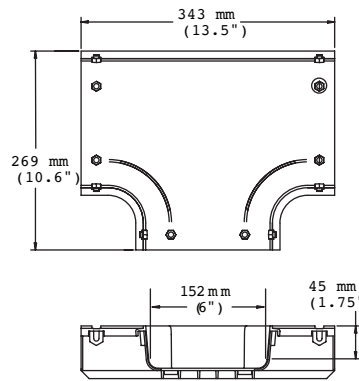
Horizontal T (FGS-MHRT-G)
